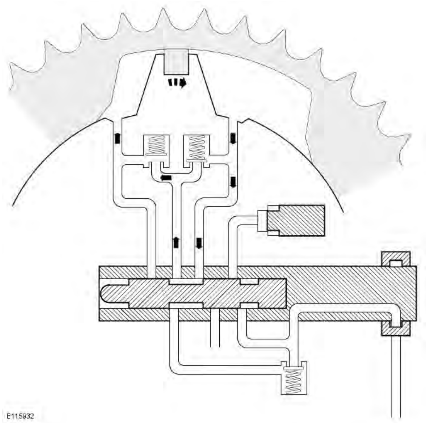
可变凸轮轴正时执行器示意图 — 提前
